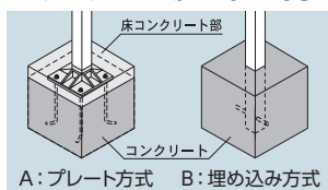
A: プレート方式 B: 埋め込み方式
