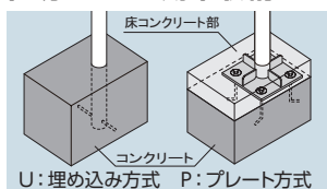
U: 埋め込み方式 P: プレート方式
